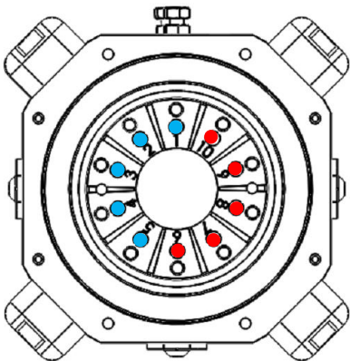
CANAIS DE SAÍDA (ROTOR)
